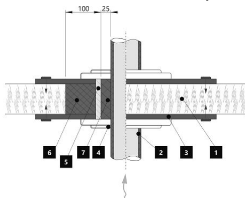
Suitsutoru läbiviik süttivast materjalist seinast
