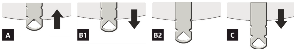
Abb. 9 Luftzufuhrregler – Typ 5
