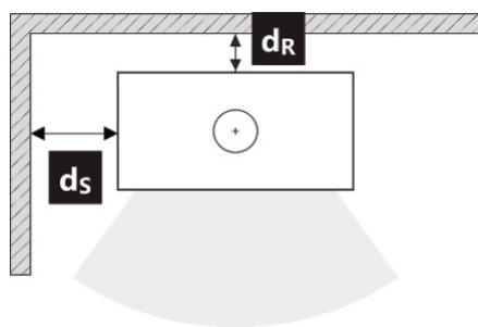
Abb. 3 Abstand zu nicht brennbaren Materialien
