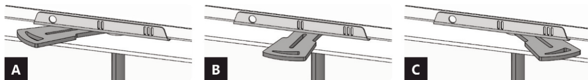
Abb. 7 Luftzufuhrregler – Typ 3
