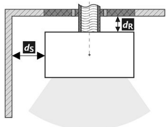
Raccordement arrière du conduit de fumée (isolé)
