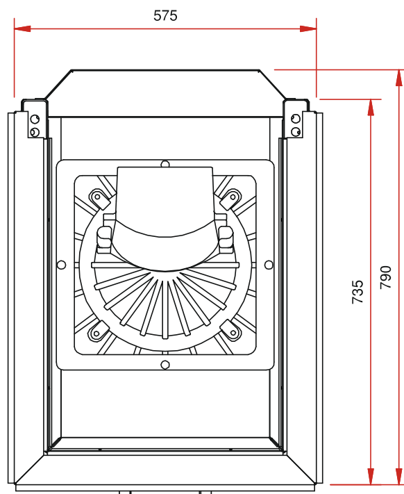
pealtvaade M 1:10
