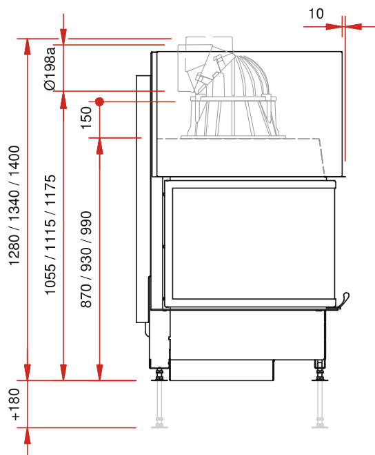
külgvaade M 1:20
