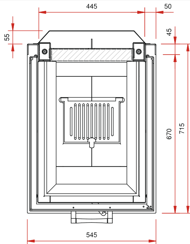
põhiplaan M 1:10
