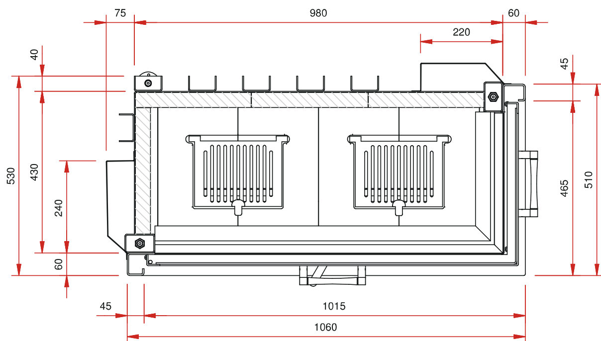
põhiplaan M 1:10
