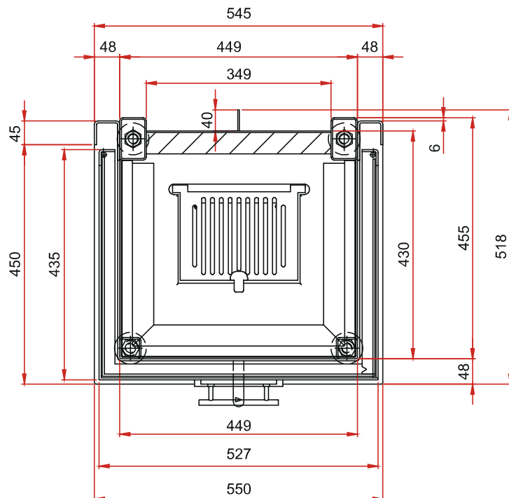
pealtvaade M 1:10
