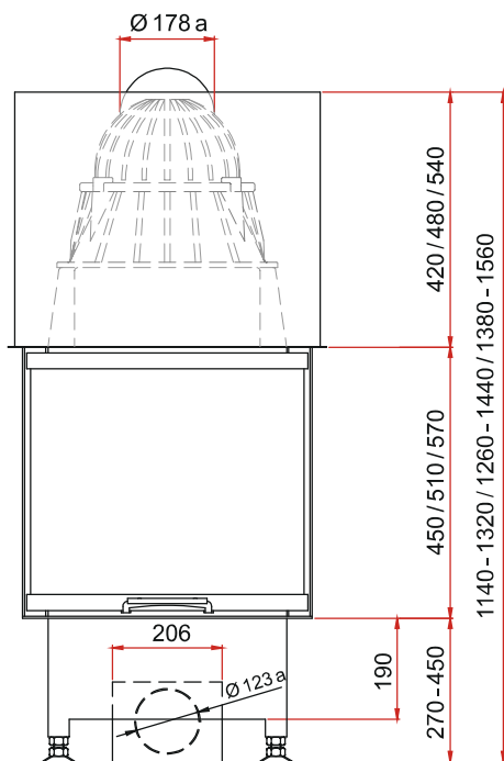
külgvaade M 1:20
