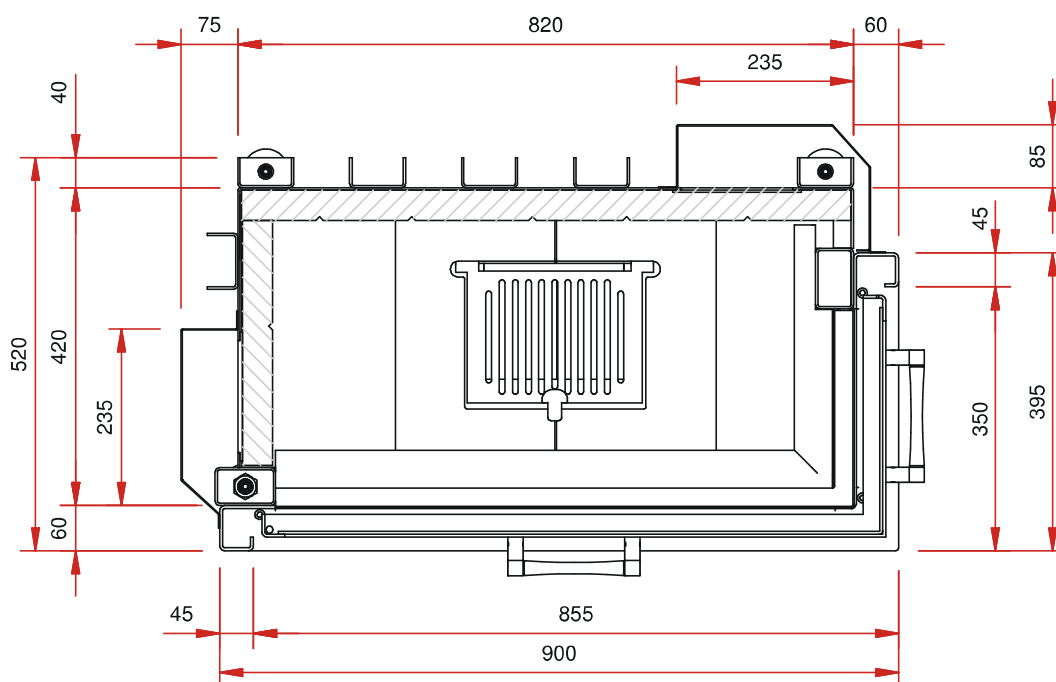
põhiplaan M 1:10
